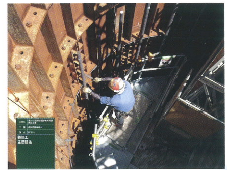
アーバンファンデーション工法の 施工状況
