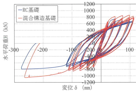
荷重－変位曲線
