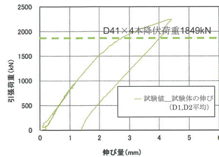
帯筋としての伸び量評価
